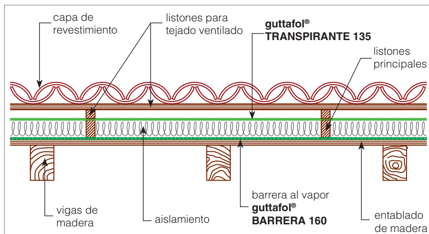
Fig. 2 guttafol® TRANSPIRANTE 135 sobre el aislamiento con cámara de ventilación
