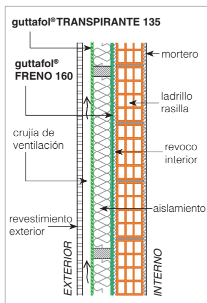
Fig. 1 guttafol® TRANSPIRANTE 135 por pared
