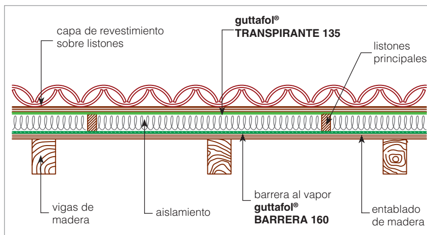
Fig. 3 guttafol® TRANSPIRANTE 135 sobre el aislamiento sin cámara de ventilación
